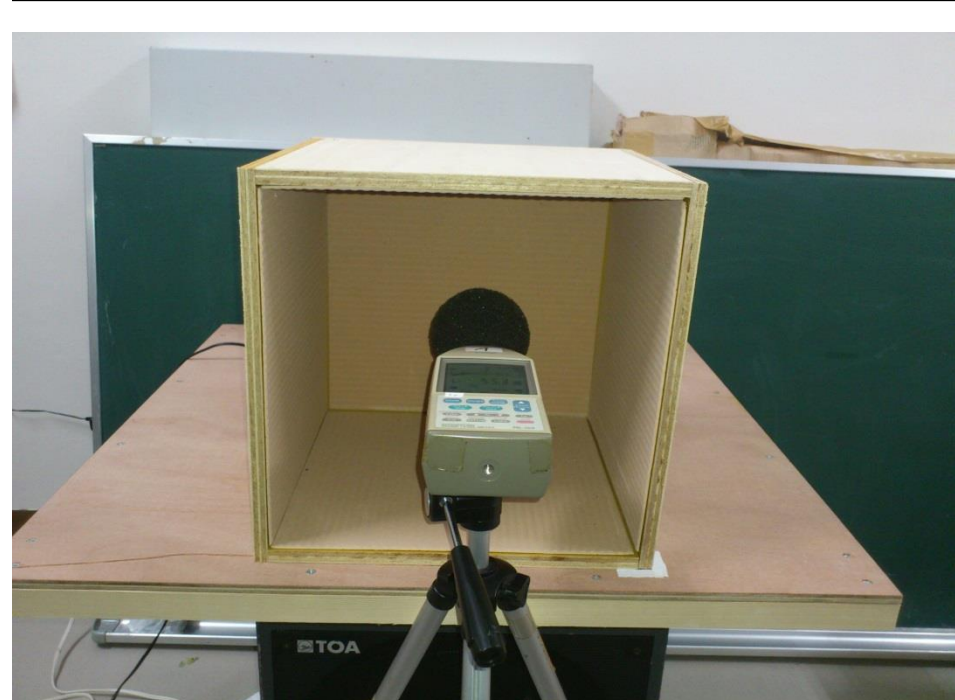
吸音材を設置
