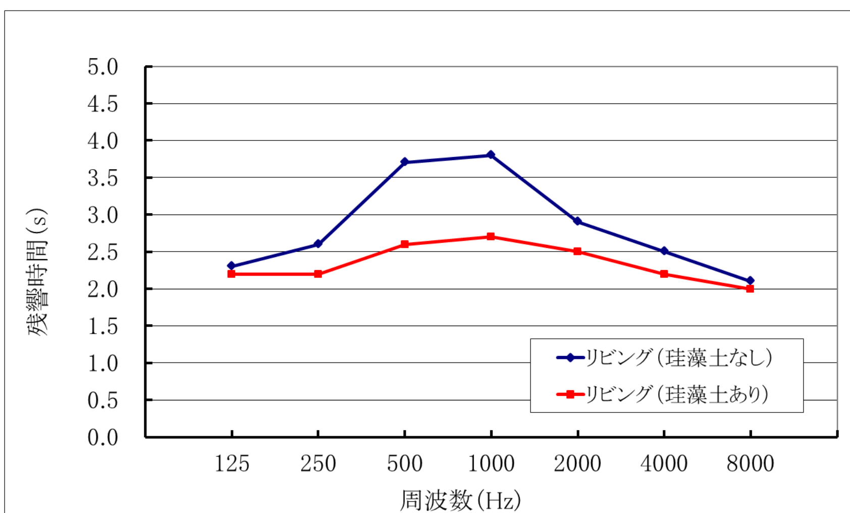
珪藻土施工前と施工後の残響時間の比較
