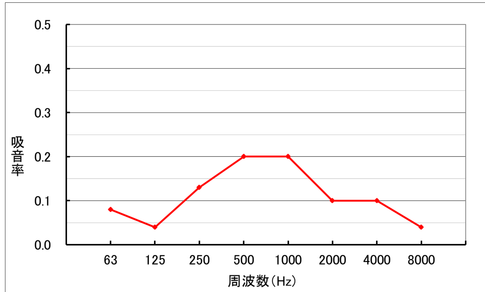
珪藻土吸音率
