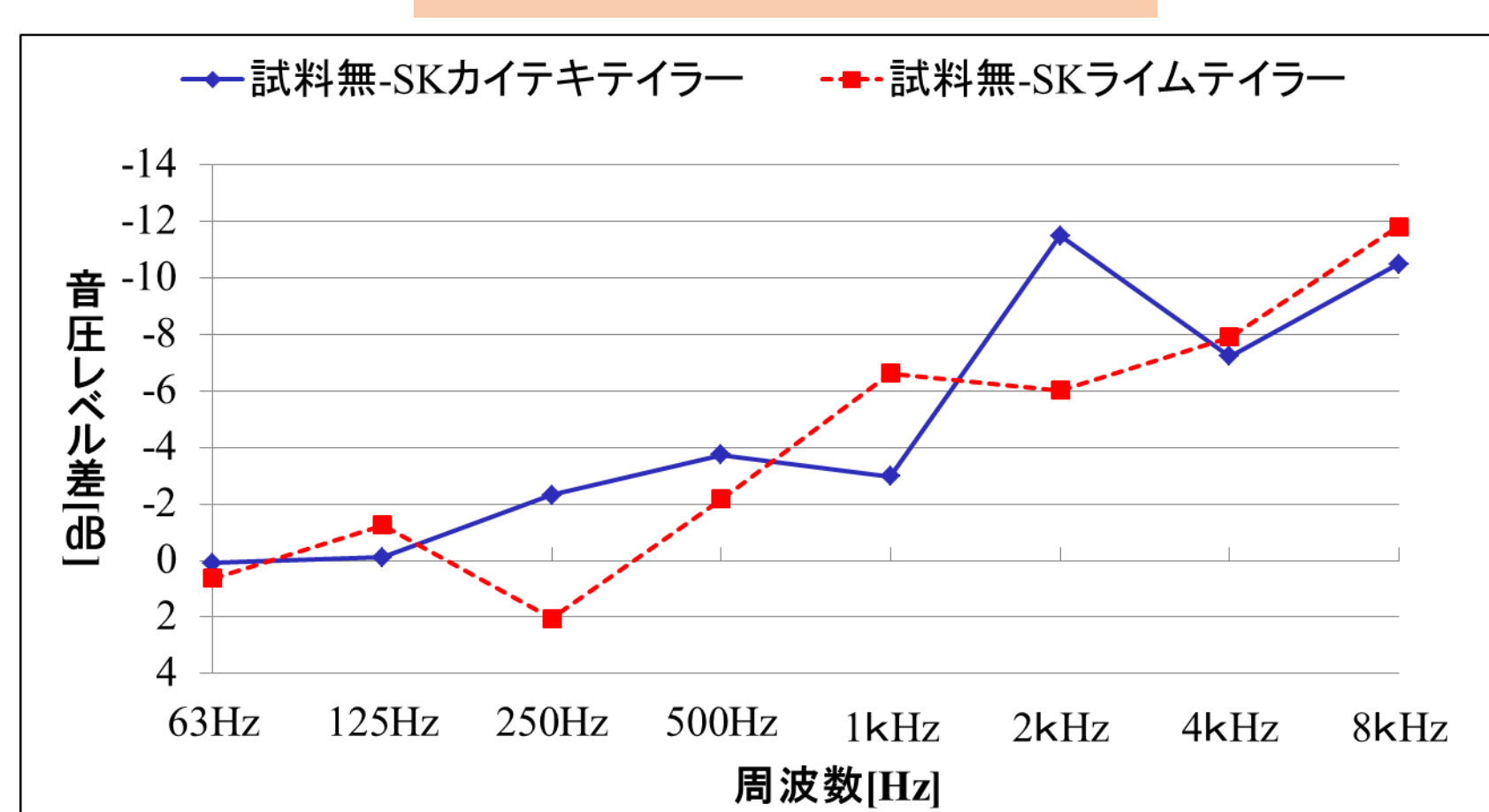
周波数別減音量
